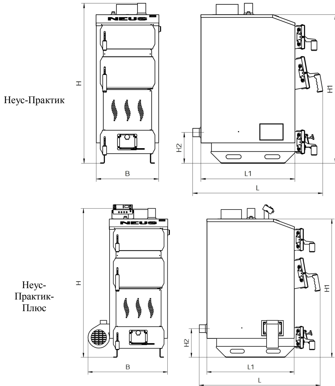
Рисунок 1 – Габаритне креслення котла Неус-Практик (Неус-Практик-Плюс)
