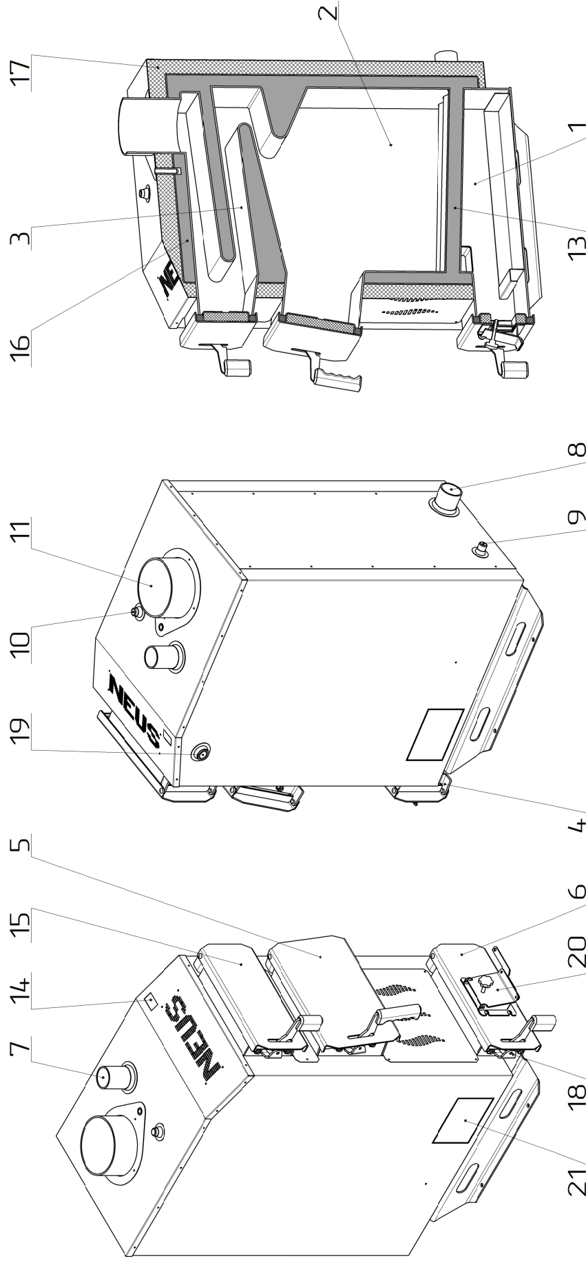
Рисунок 2а – Основні елементи котла Неус-Практик
