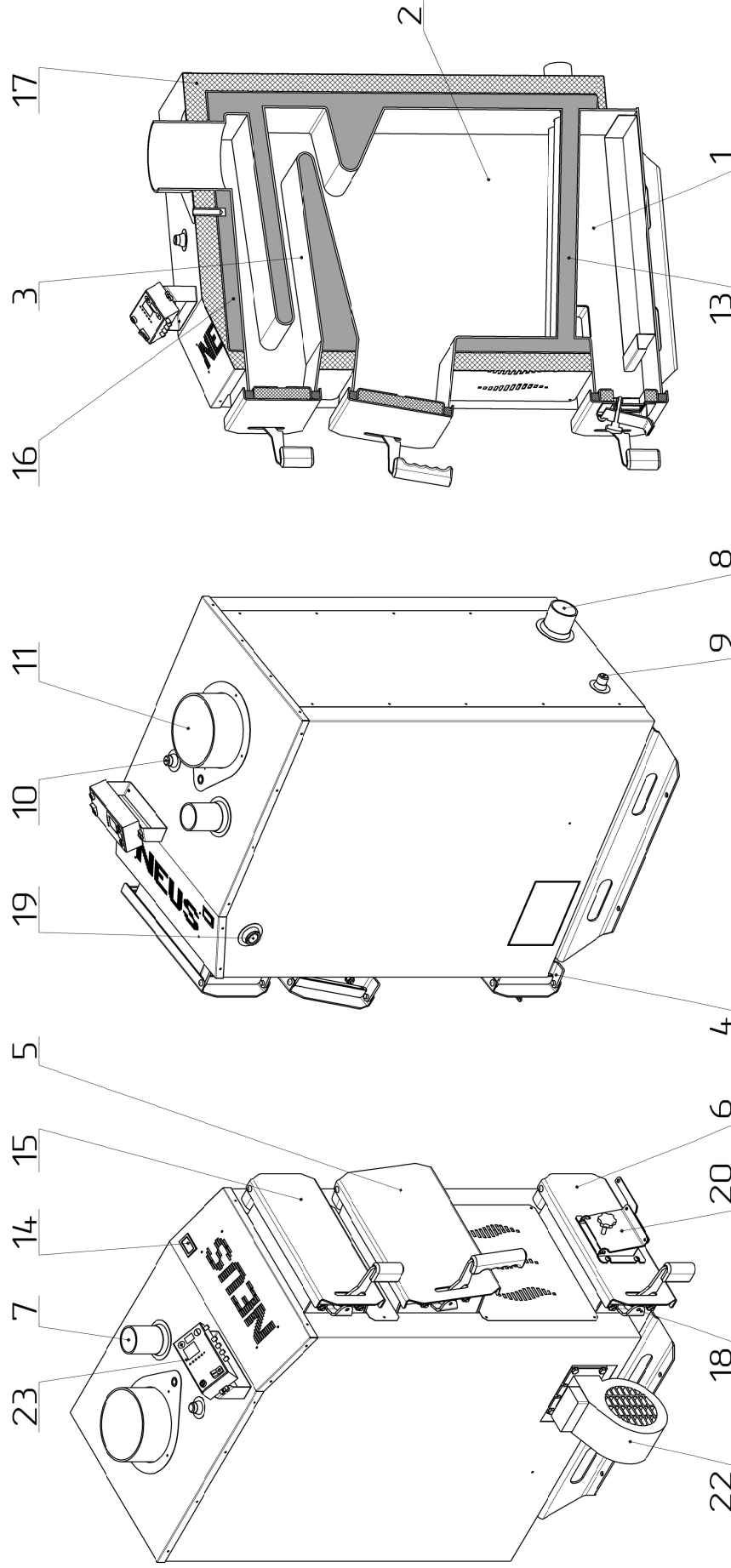
Рисунок 2б – Основні елементи котла Неус-Практик-Плюс
